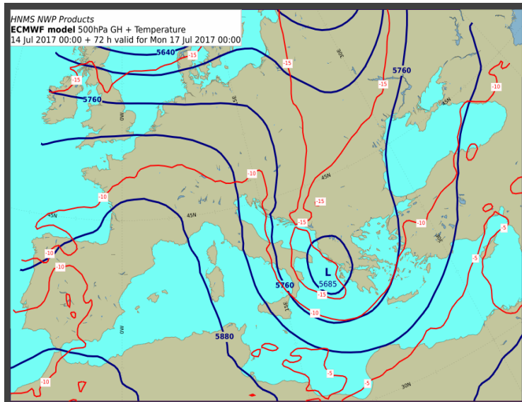
Σχήμα 1. 500 hpa: ισουψείς ανά 60 gpm (μπλε γραμμές), ισόθερμες ανά 5°C (κόκκινες γραμμές)
