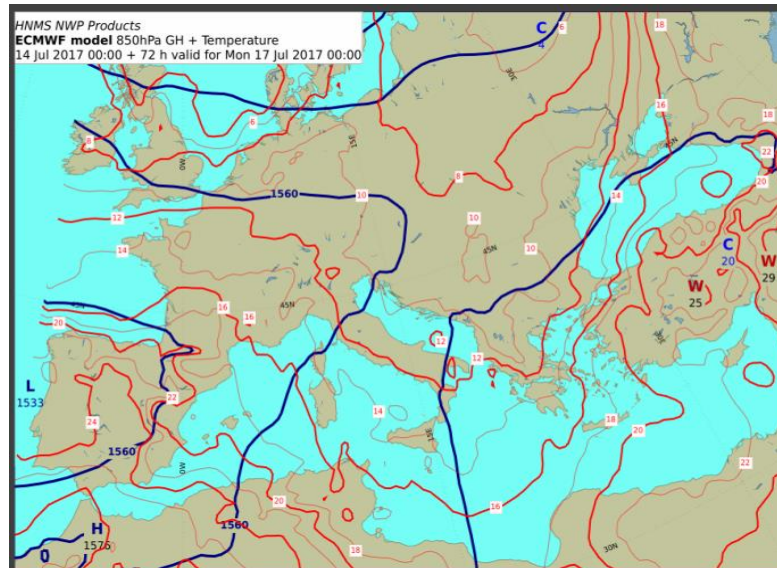
Σχήμα 3. 850 hpa: ισουψείς ανά 60 gpm (μπλε γραμμές), ισόθερμες ανά 2°C (κόκκινες γραμμές)
